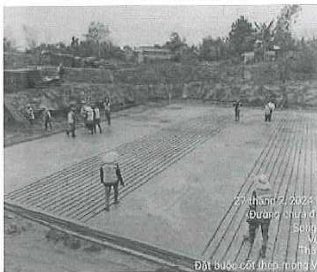
Xây lắp đường dây đoạn tuyến từ VT141 đến VT151 (bao gồm VT151) thuộc dự án: đường dây 500kv NMND Nam Định I – Phố Nối.
