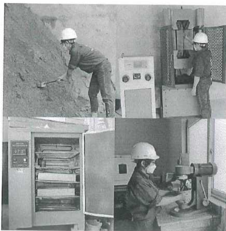
Kiểm tra chất lượng nguyên vật liệu
