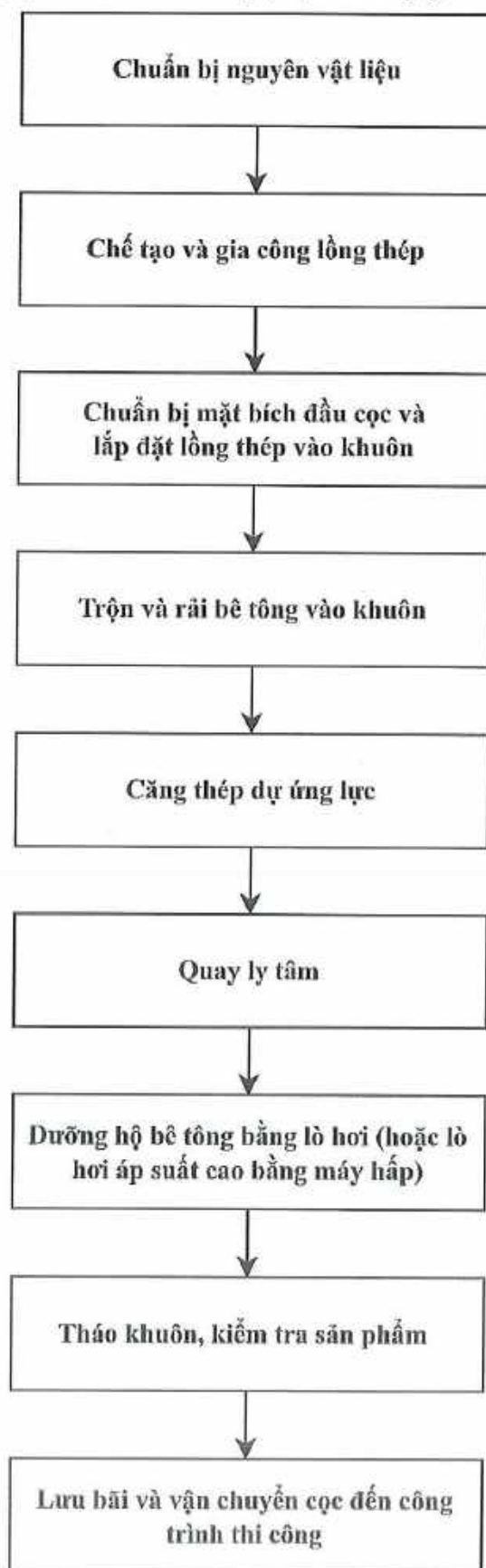
Hình 10. Quy trình sản xuất cọc, cột bê tông ly tâm dự ứng lực
