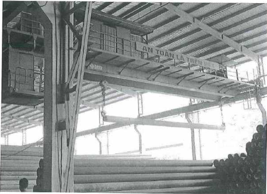
Bước 9: Lưu bãi và vận chuyển cọc đến công trình thi công.
