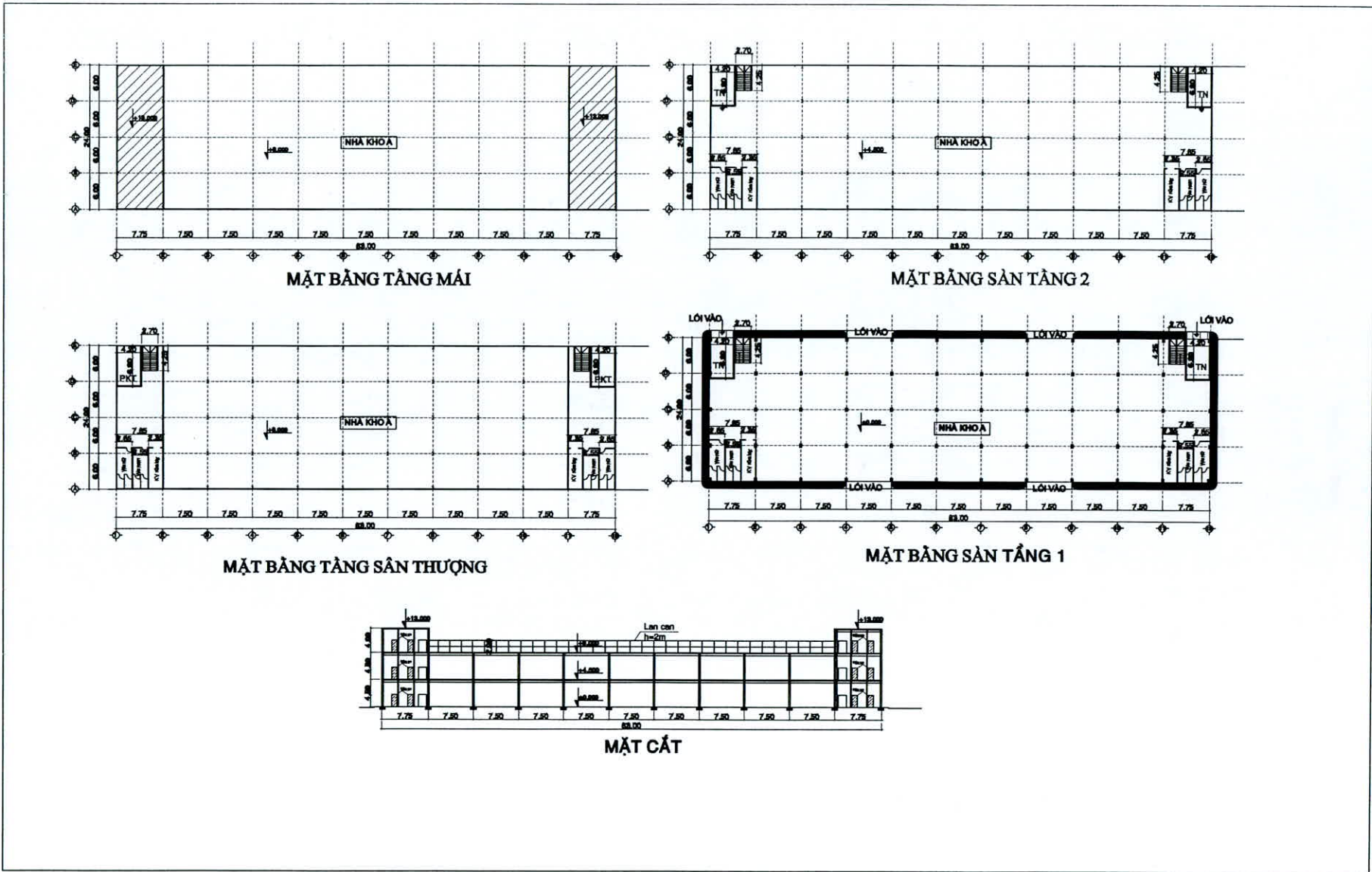
MẶT BẰNG NHÀ KHO A CẢI TẠO (NHỊP 6M)
